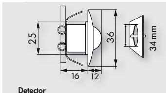
Detector
